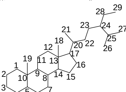
甾类
