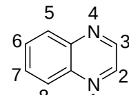
喹喔啉
