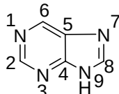
嘌呤
