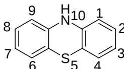
吩噻嗪
