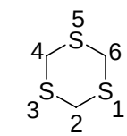
1,3,5-三噻烷
