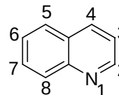
喹啉
