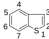
苯并[b]噻吩
