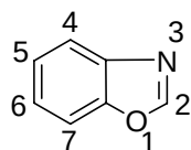
苯并恶唑
