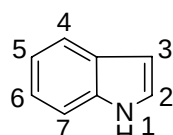
吲哚
