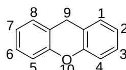
氧杂蒽
