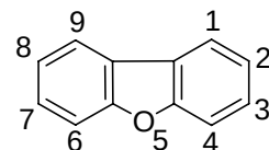
二苯并呋喃
