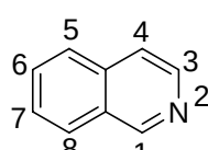
异喹啉
