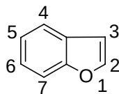
苯并呋喃
