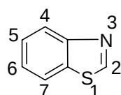
苯并噻唑
