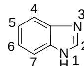
苯并咪唑
