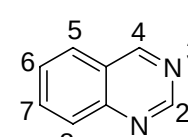
喹唑啉
