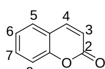
香豆素
