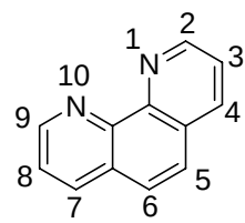
1,10-菲咯啉
